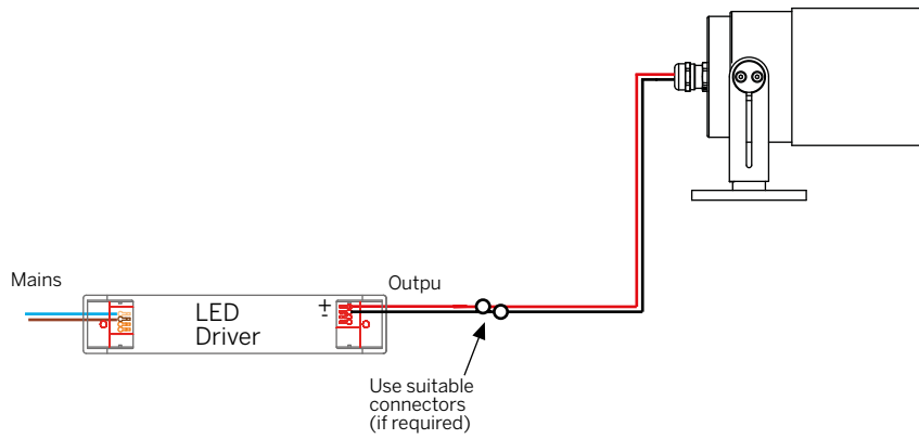
Croc Wiring
